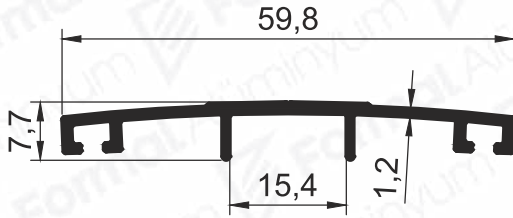
Pr.No: 9328 0,305 kg/m
