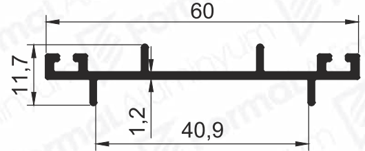
Pr.No: 9327 0,313 kg/m
