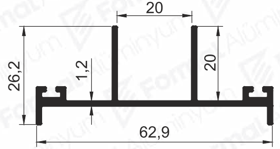
Pr.No: 9369 0,459 kg/m
