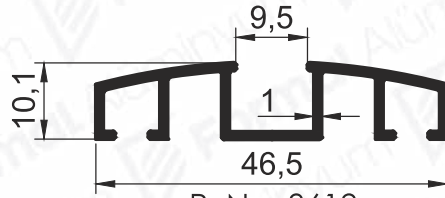
Pr.No: 8612 0,275 kg/m
