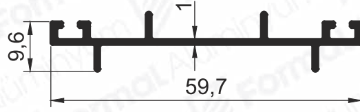
Pr.No: 3823 0,273 kg/m
