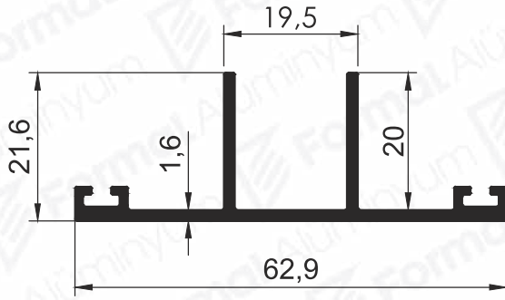
Pr.No: 9370 0,521 kg/m
