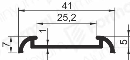
Pr.No: 8726 0,172 kg/m
