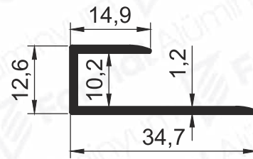
Pr.No: 2241 0,189 kg/m
