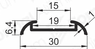
Pr.No: 9277 0,121 kg/m
