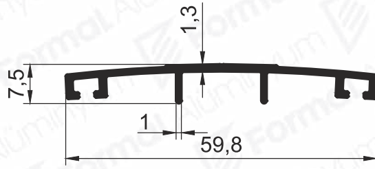
Pr.No: 3824 0,281 kg/m
