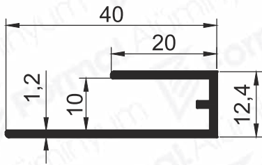
Pr.No: 5269 0,235 kg/m
